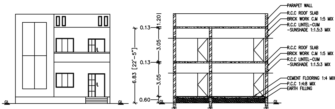
ELEVATION
