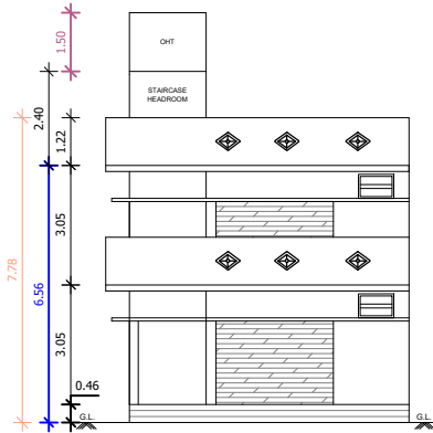
ELEVATION-A
