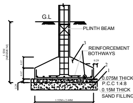
TYP. DET. COLUMN FOOTING
