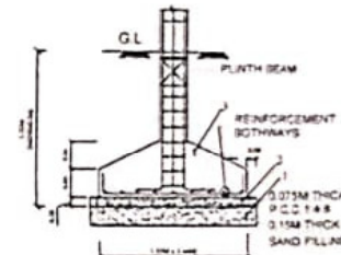
TYP. DET. COLUMN FOOTING
