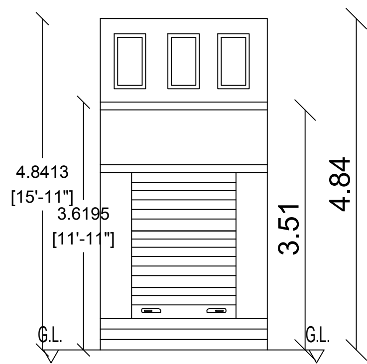
ELEVATION
