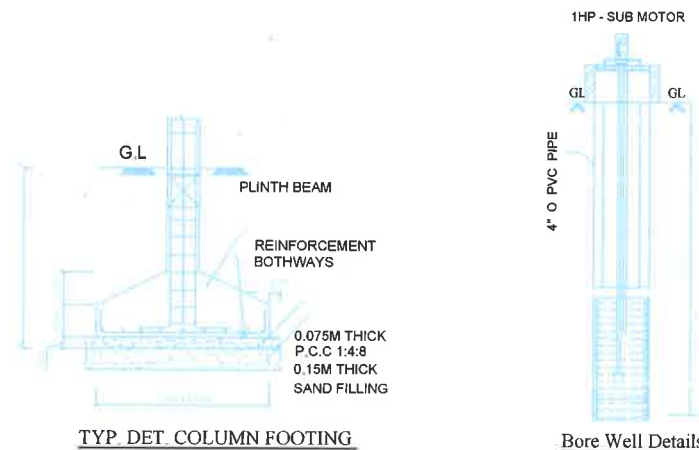
TYP. DET. COLUMN FOOTING
