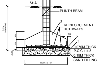
TYP. DET. COLUMN FOOTING
