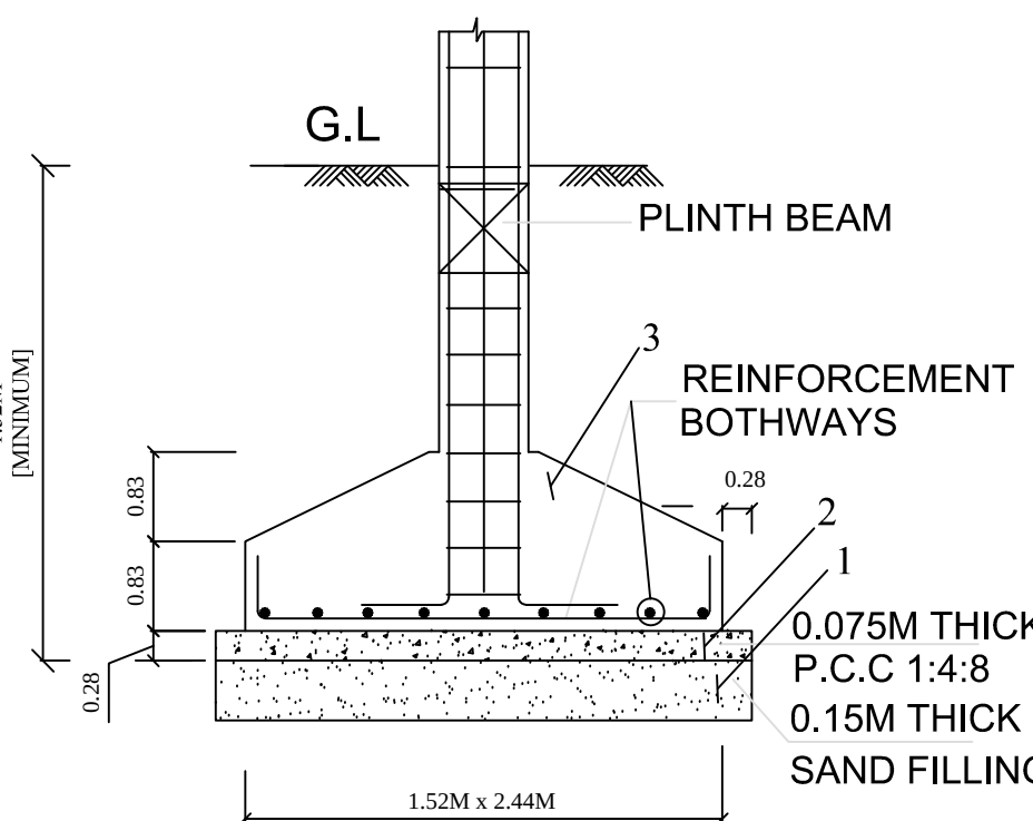
TYP. DET. COLUMN FOOTING
