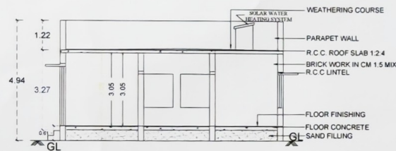
SECTION A-B
