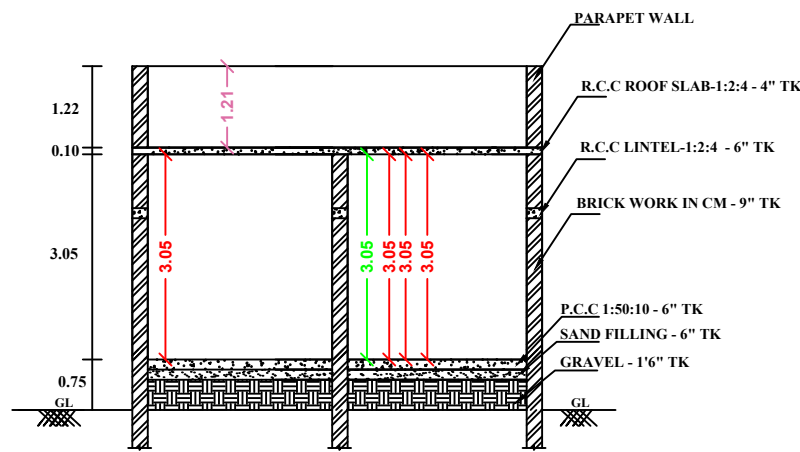
SECTION - AB
