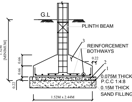
TYP. DET. COLUMN FOOTING
