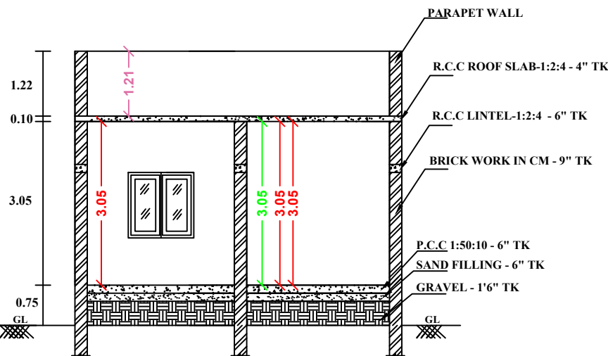
SECTION -AB
