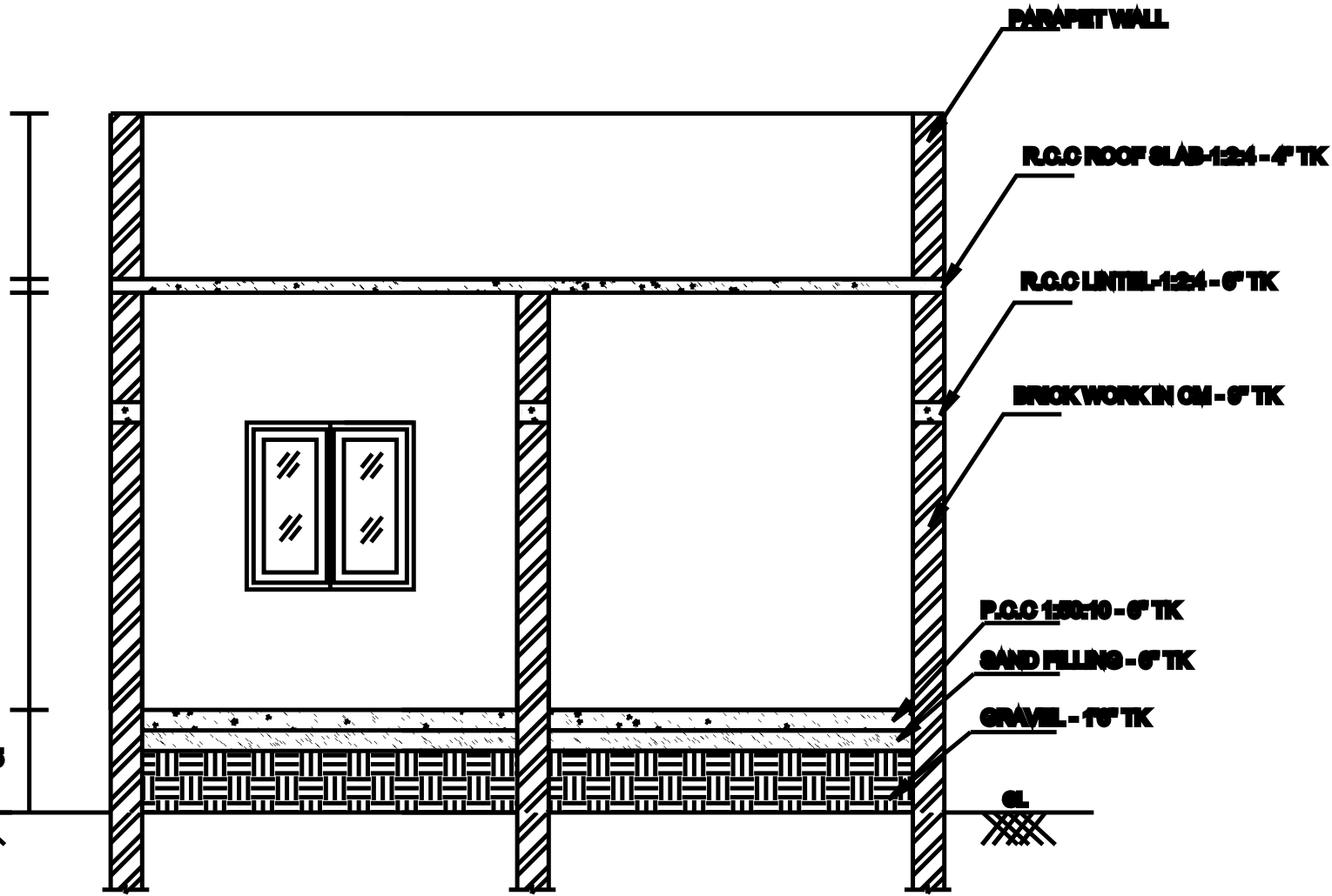
SECTION -AB
