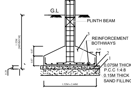
TYP. DET. COLUMN FOOTING
