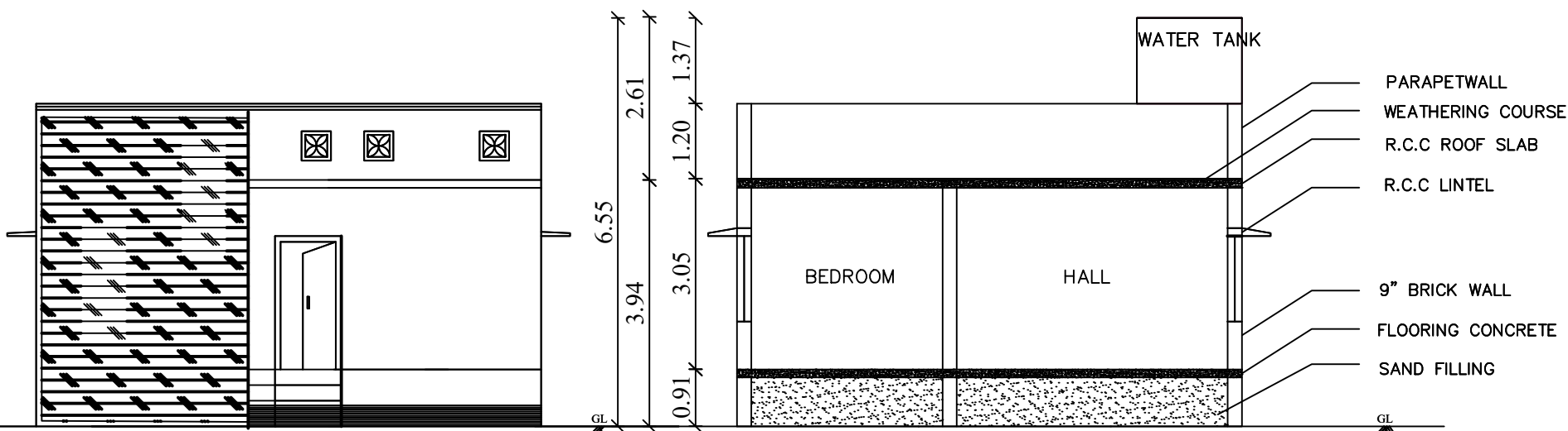
ELEVATION
