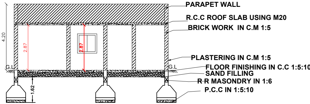
SECTION A-A PLOT NO:8 12.37
