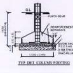
TYP DET. COLUMN FOOTING
