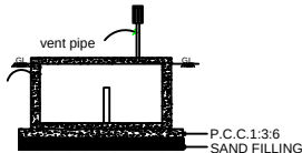
SECTION ON DD SCALE 1:100
