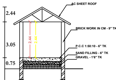
SECTION -AB
