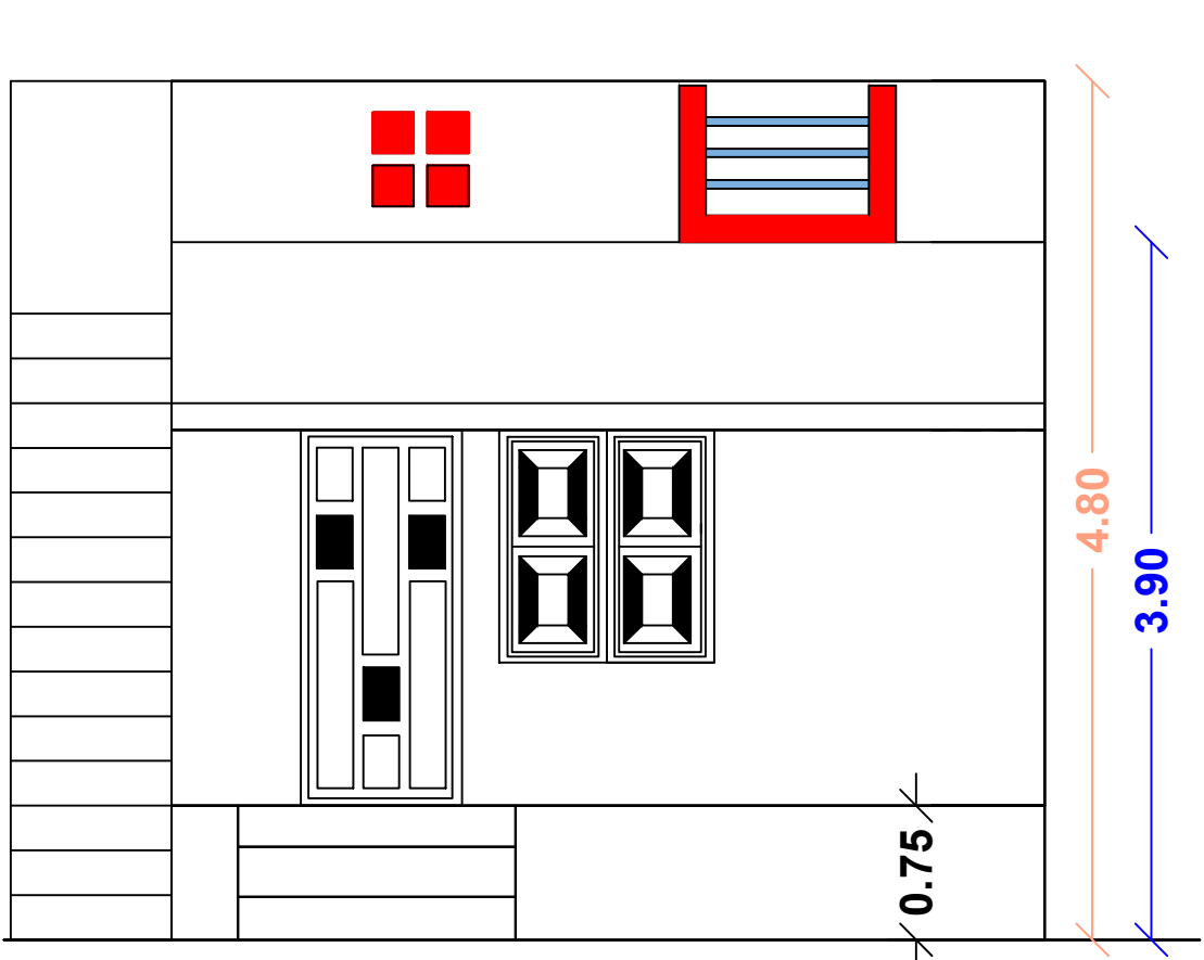
ELEVATION
