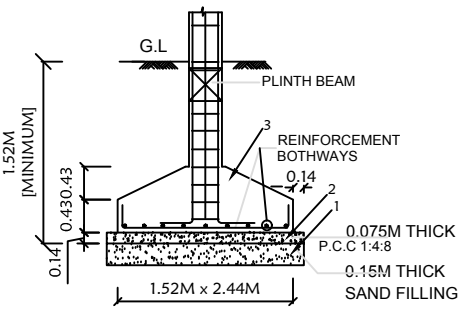
TYP. DET. COLUMN FOOTING
