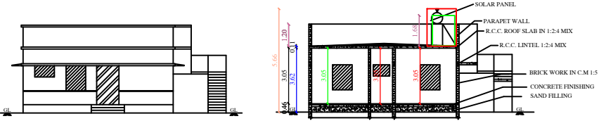
ELEVATION
