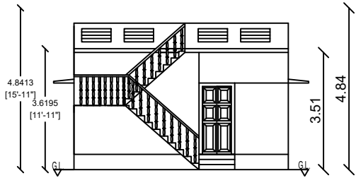
ELEVATION
