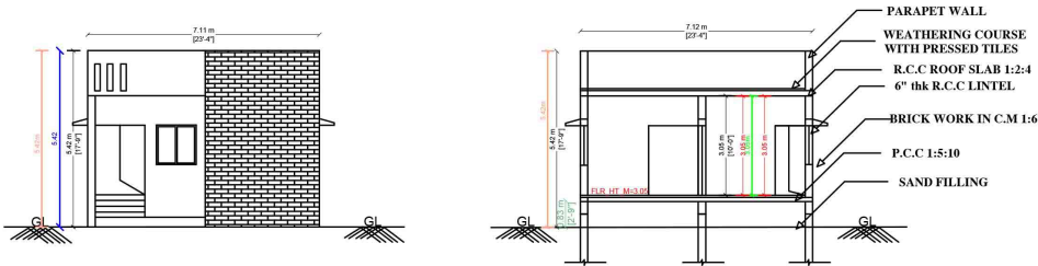
ELEVATION
