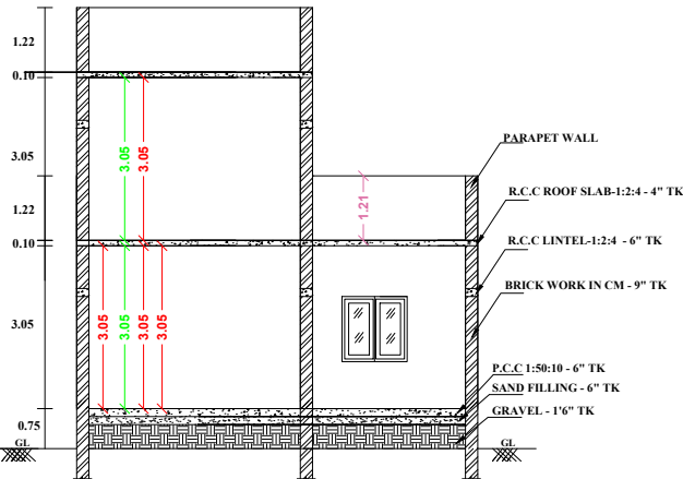
SECTION -AB
