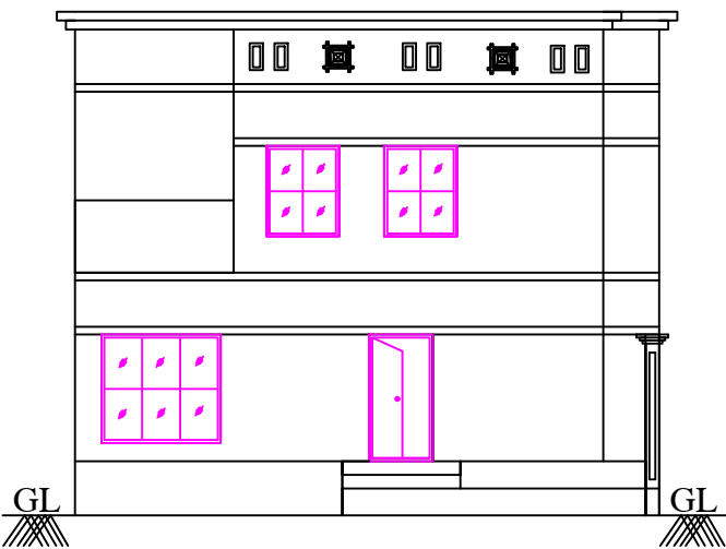
ELEVATION
