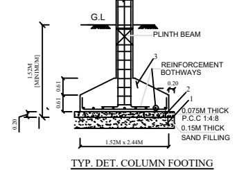
TYP. DET. COLUMN FOOTING
