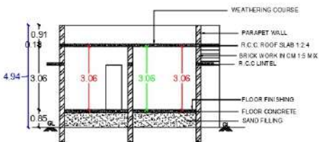
SECTION A-B
