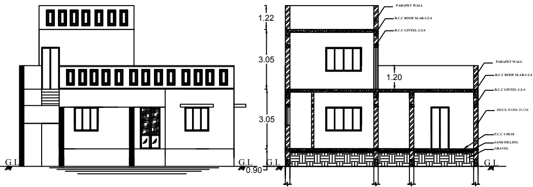
ELEVATION
