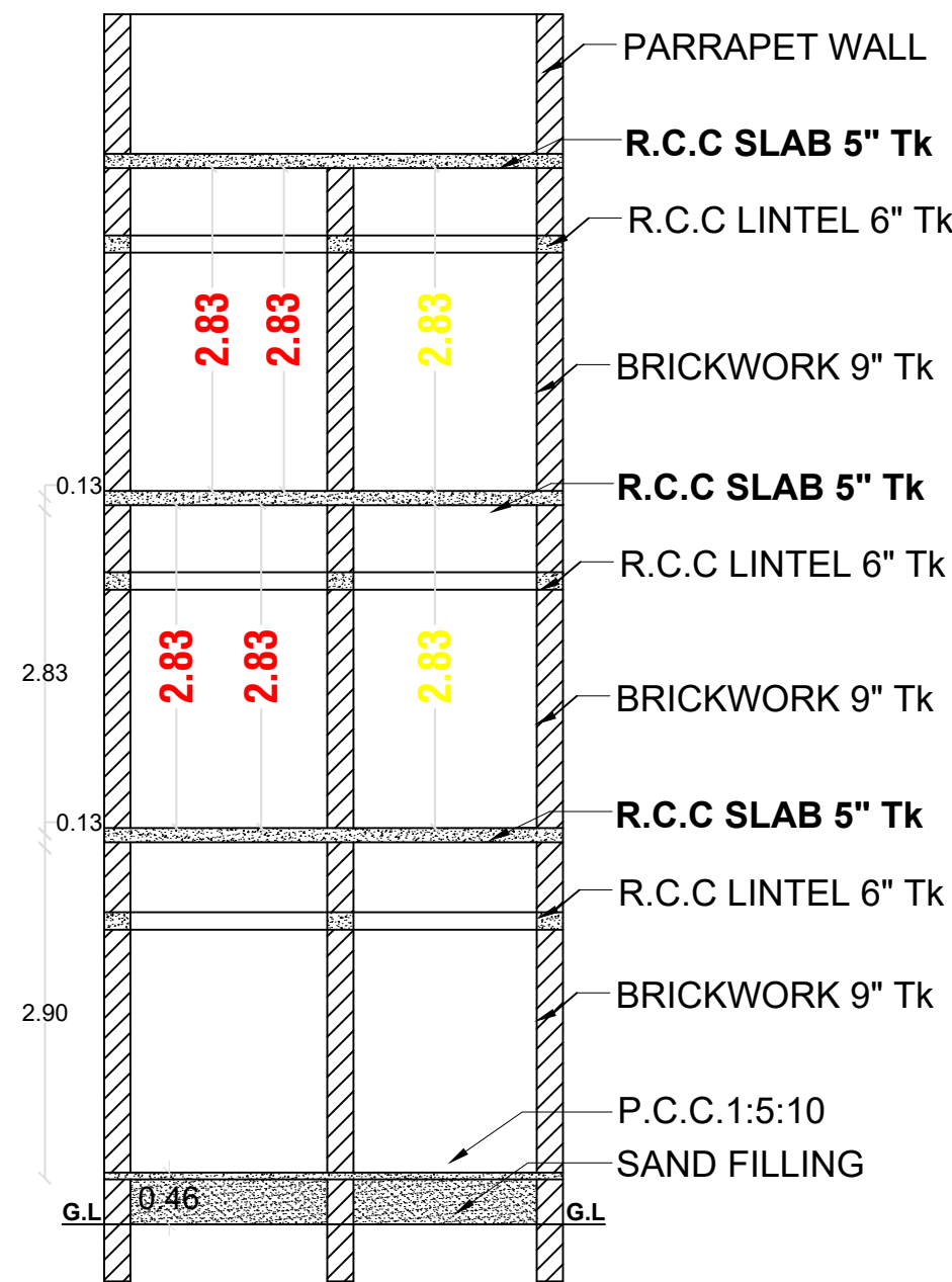
SECTION A-A'
