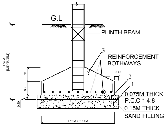
TYP. DET. COLUMN FOOTING
