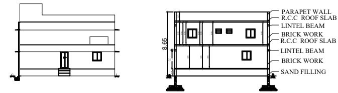
ELEVATION
