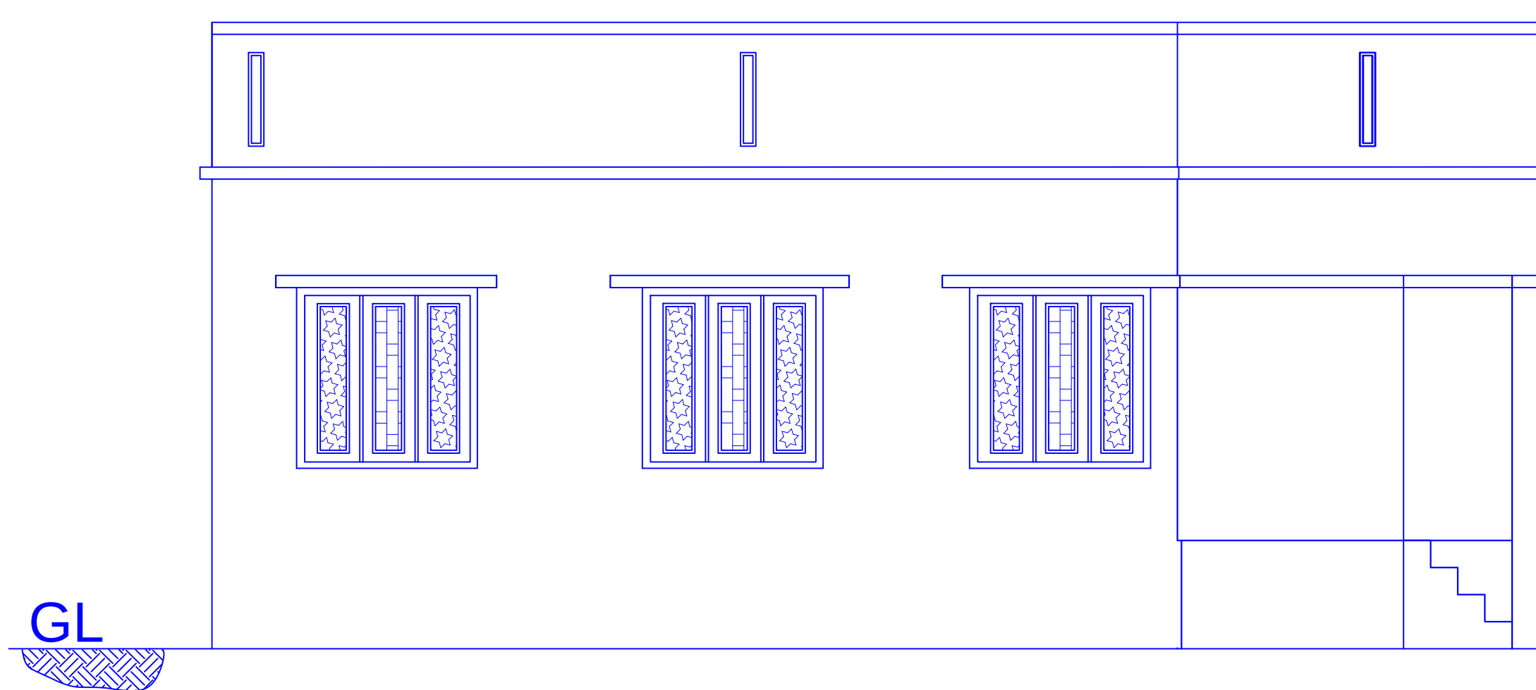
ELEVATION
