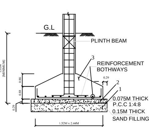
TYP. DET. COLUMN FOOTING
