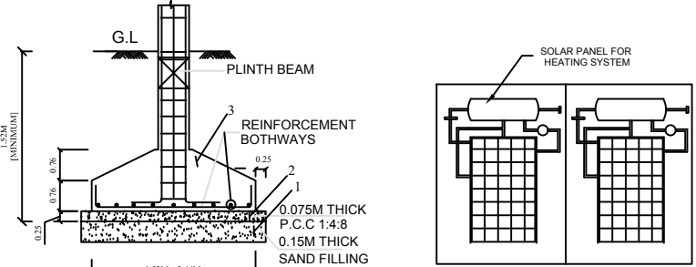
TYP. DET. COLUMN FOOTING
