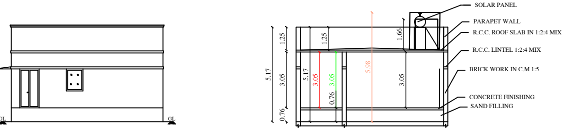
ELEVATION
