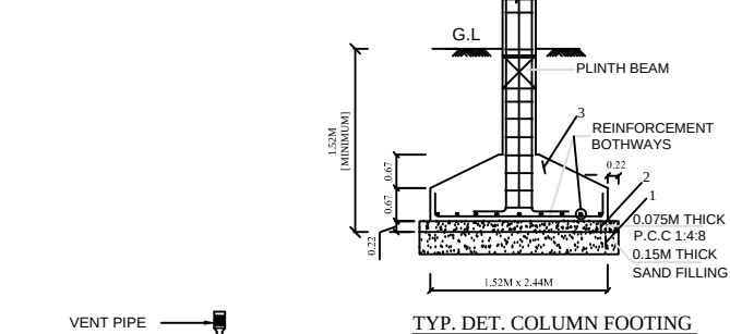
TYP. DET. COLUMN FOOTING
