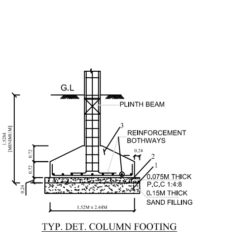
TYP. DET. COLUMN FOOTING
