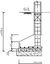
TYP. DET. COL
