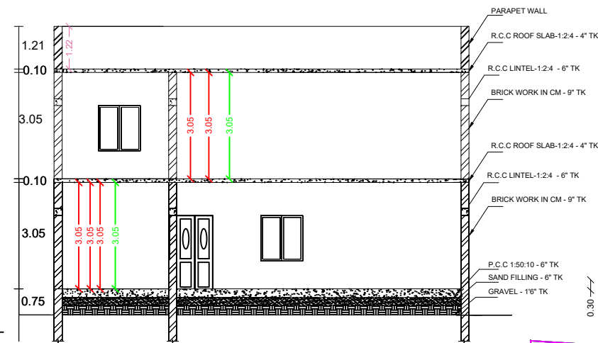
SECTION A-B
