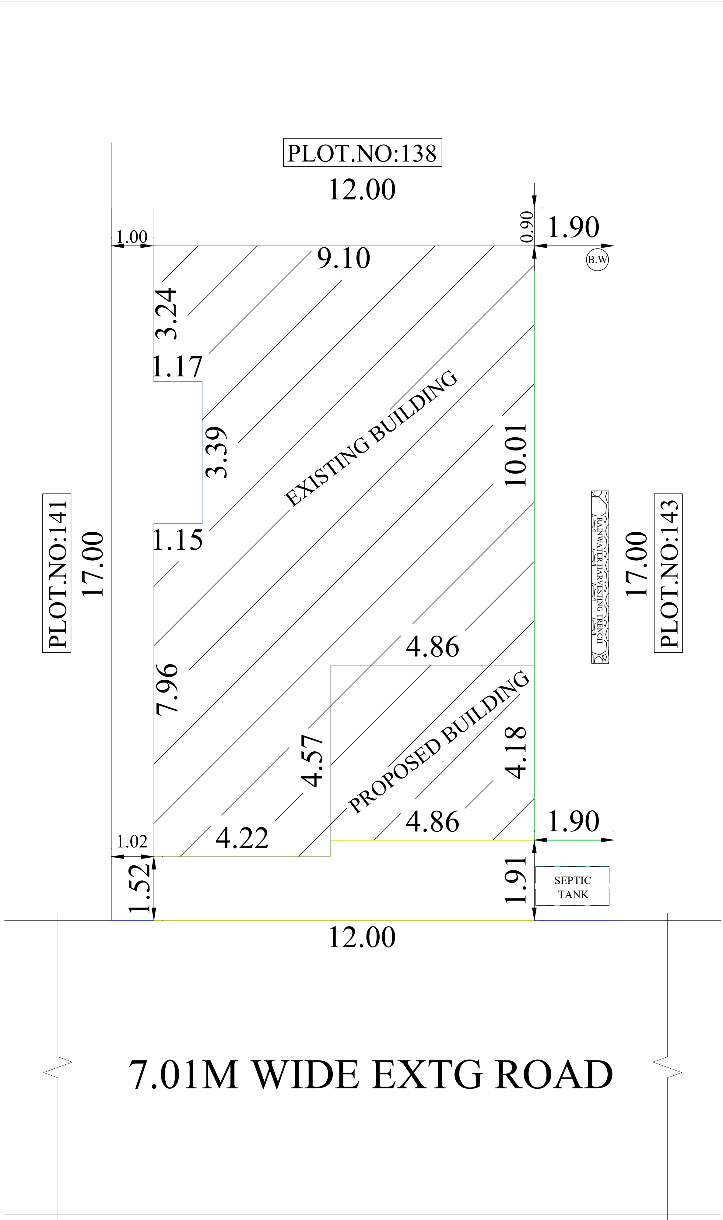
SITE PLAN 1:100
