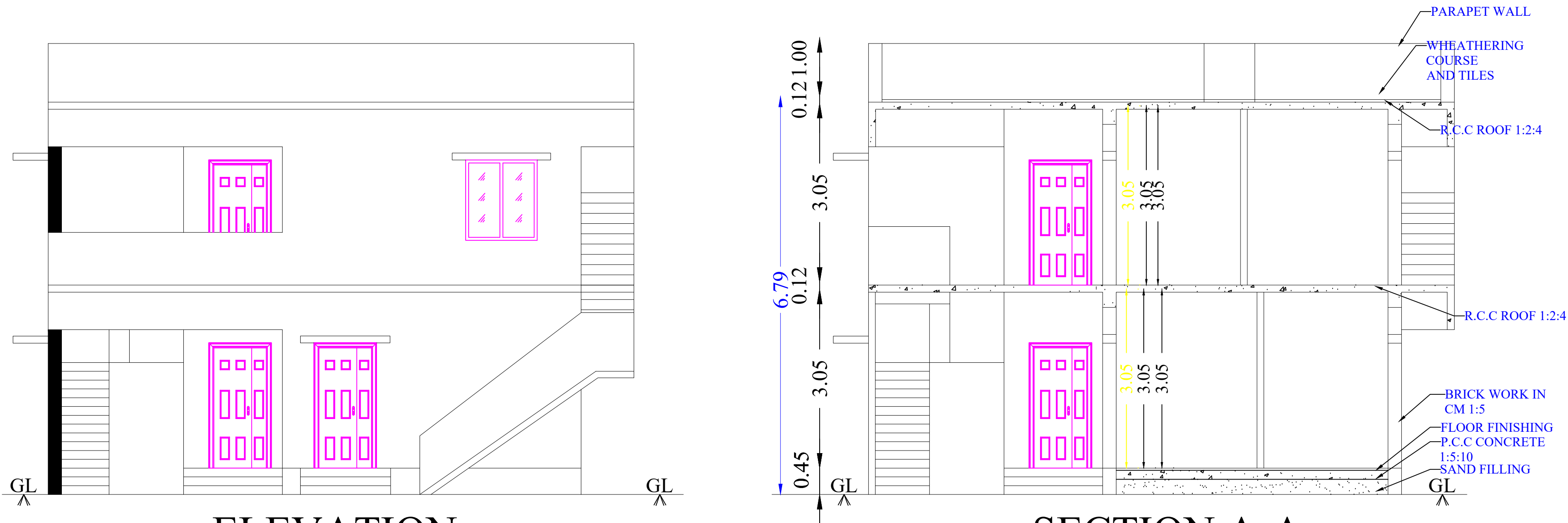
ELEVATION
