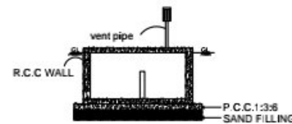
SECTION ON DD
