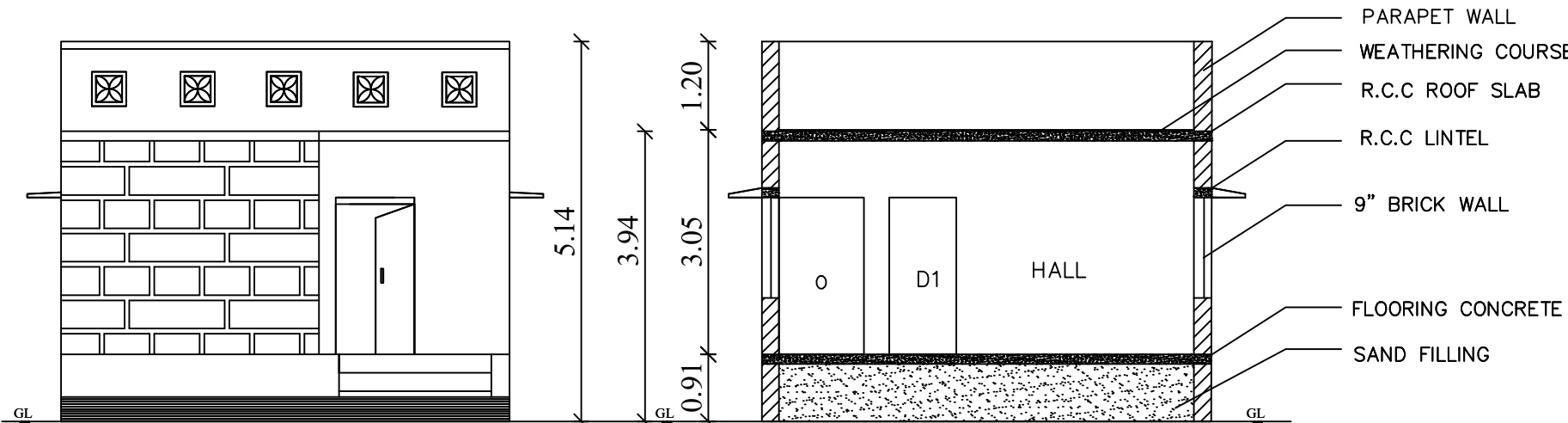
ELEVATION
