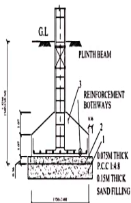
TYP. DET. COLUMN FOOTING
