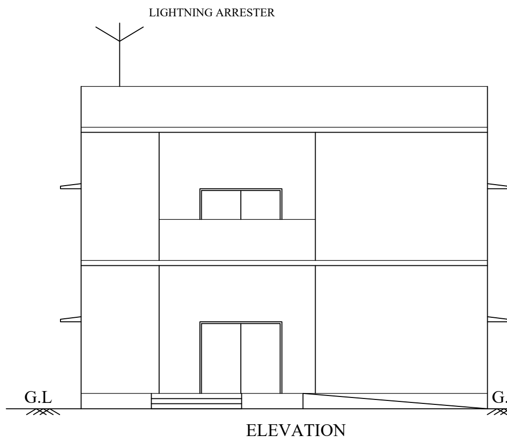
ELEVATION
