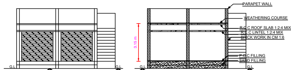
ELEVATION
