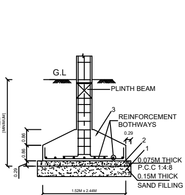
TYP. DET. COLUMN FOOTING
