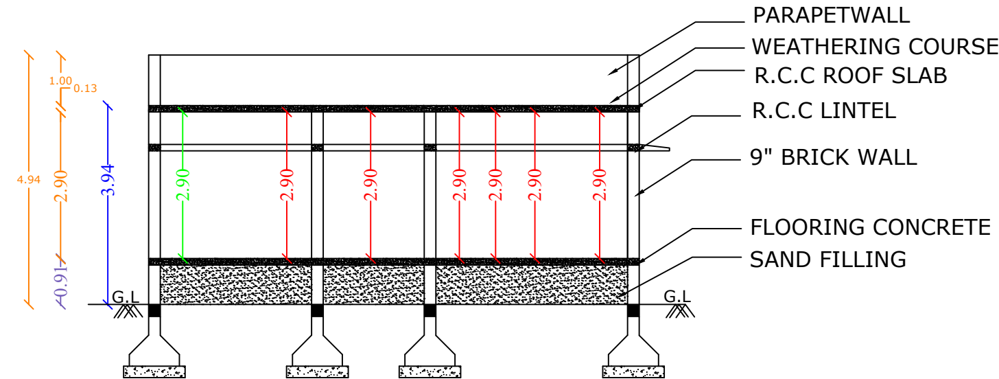
SECTION A-A'
