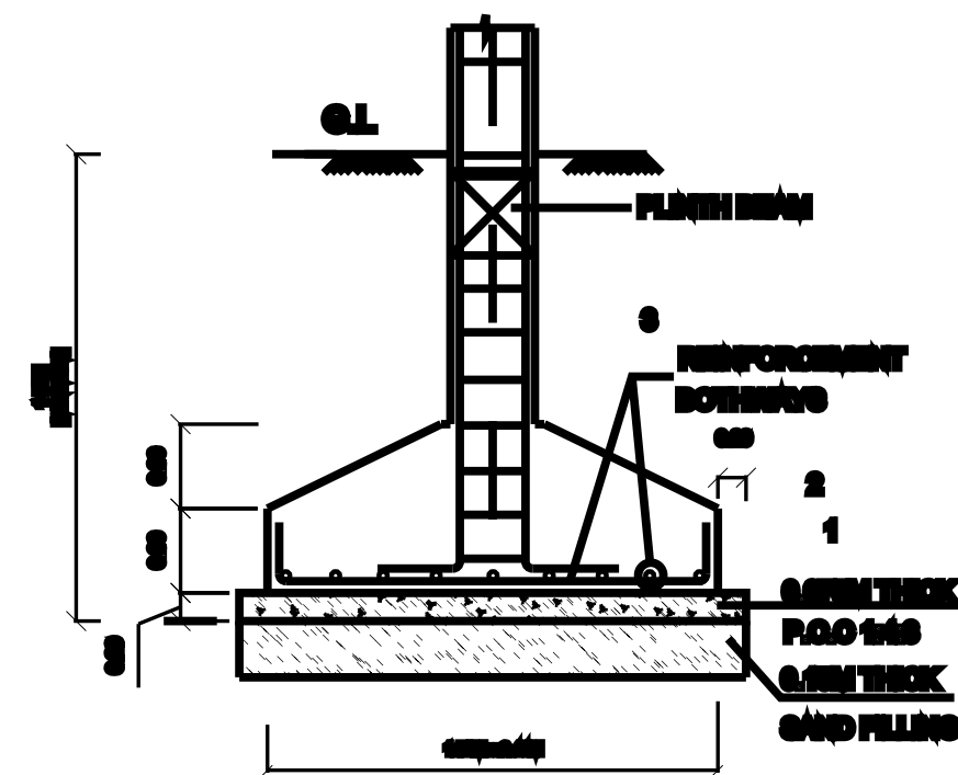
TYP. DET. COLUMN FOOTING
