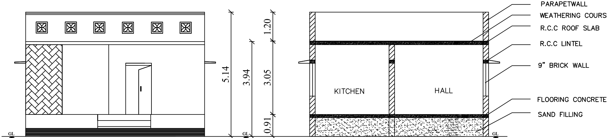
ELEVATION
